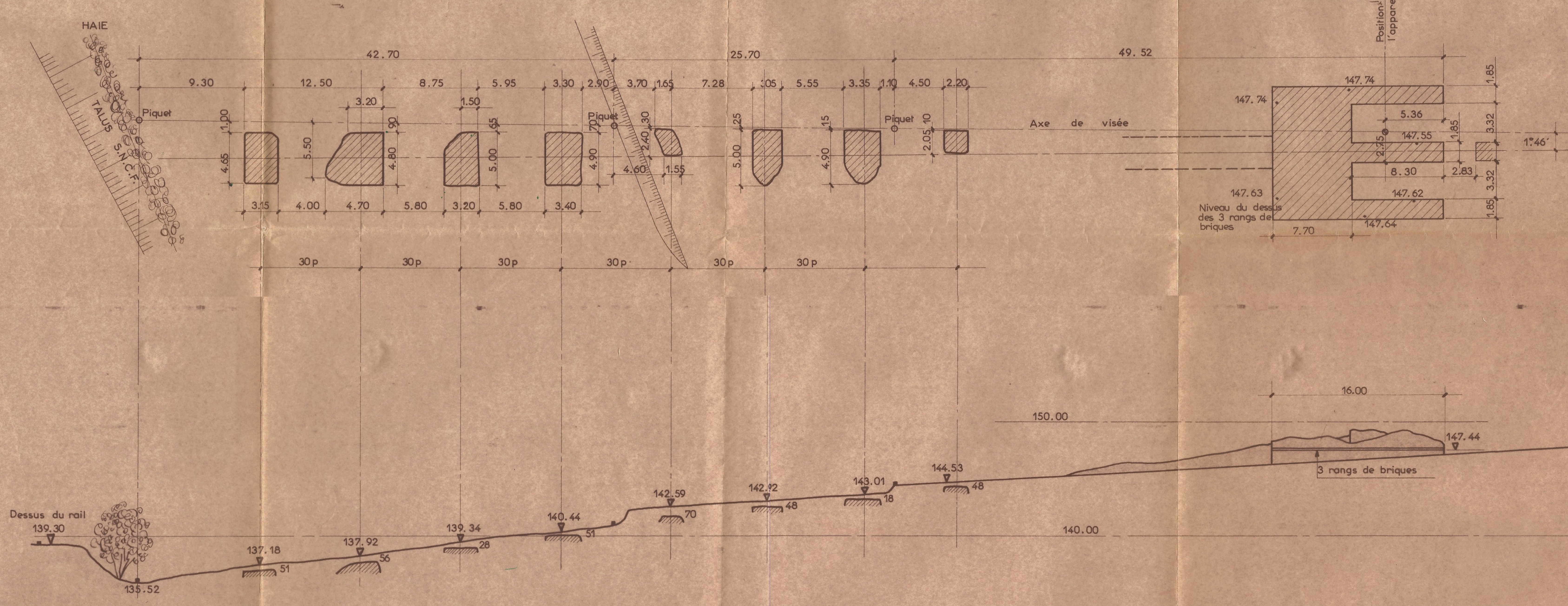
PILES DU PONT ET BASSIN DE CHARGE
