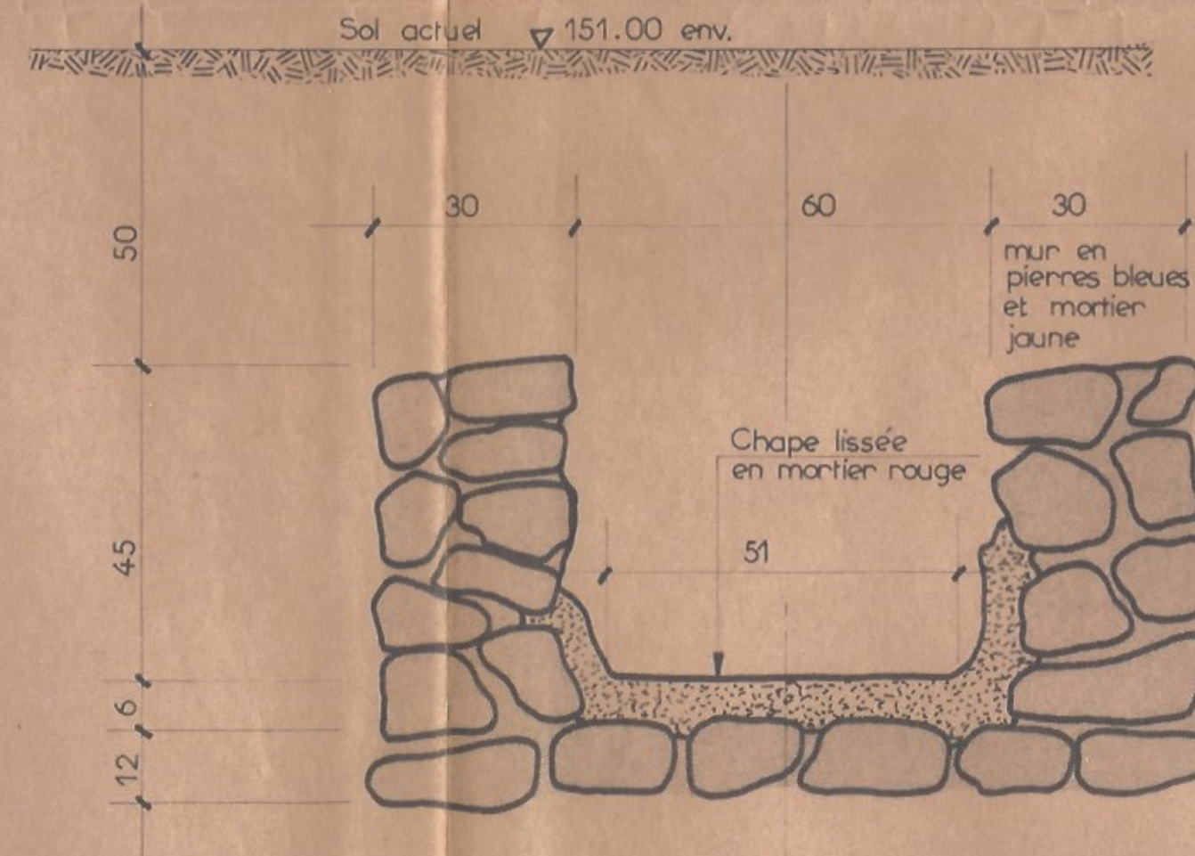
COUPE TYPE III .BAVAI.
